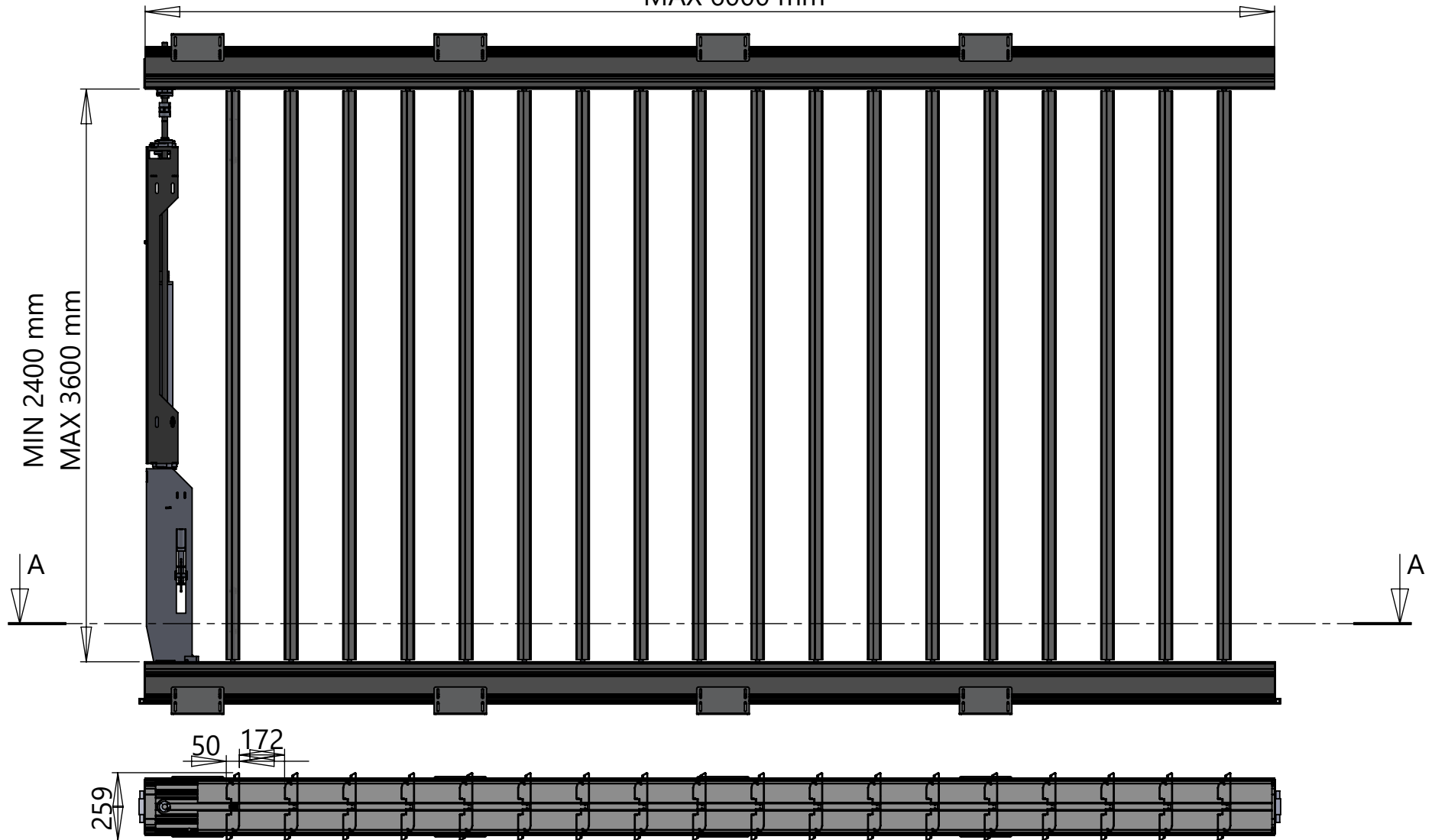
SECTION A-A
